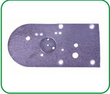
名称: 套结机针板 Description: Needle Plate 代码/Part No:10014298 适配: ZJ1900DSS Machine Type: ZJ1900DSS
