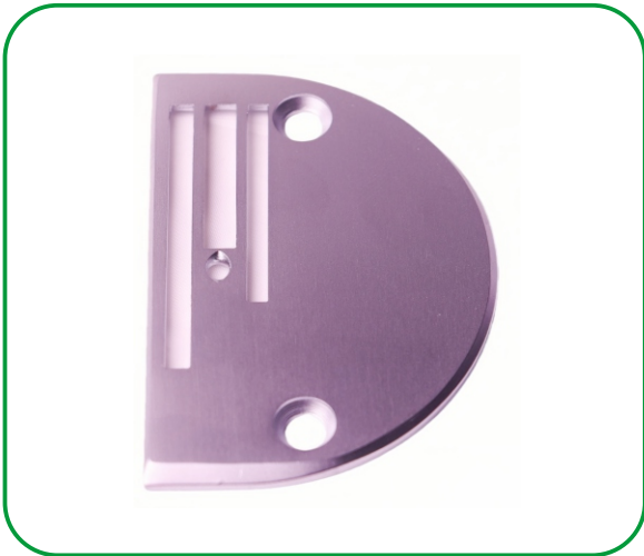
名称: 厚料针板 Description: Needle Plate 代码/Part No: 10052350 适配: ZJ8000E-D4J-H/ZJ8100E-D4J-H Machine Type: ZJ8000E-D4J-H/ZJ8100E-D4J-H
