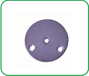
名称: 花样机小针板 Description: Needle Plate 代码/Part No:10000750 适配: ZJ5770A Machine Type: ZJ5770A
