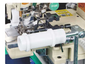
可调式松紧支架 Adjustable tension bracket
